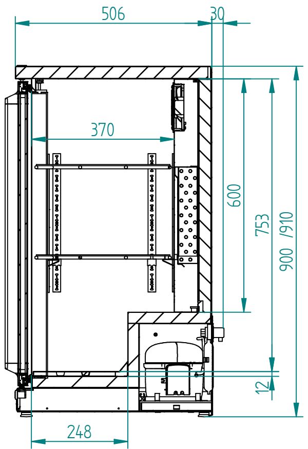
SECTION A-A
