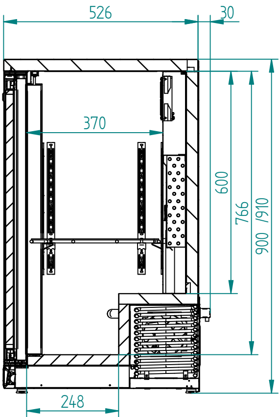
SECTION D-D
